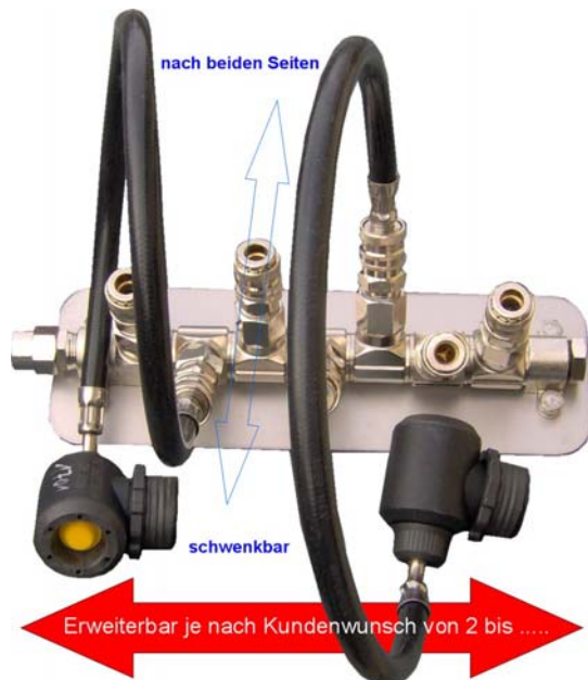
Abbildung Atemluftkonsole ALK 7
